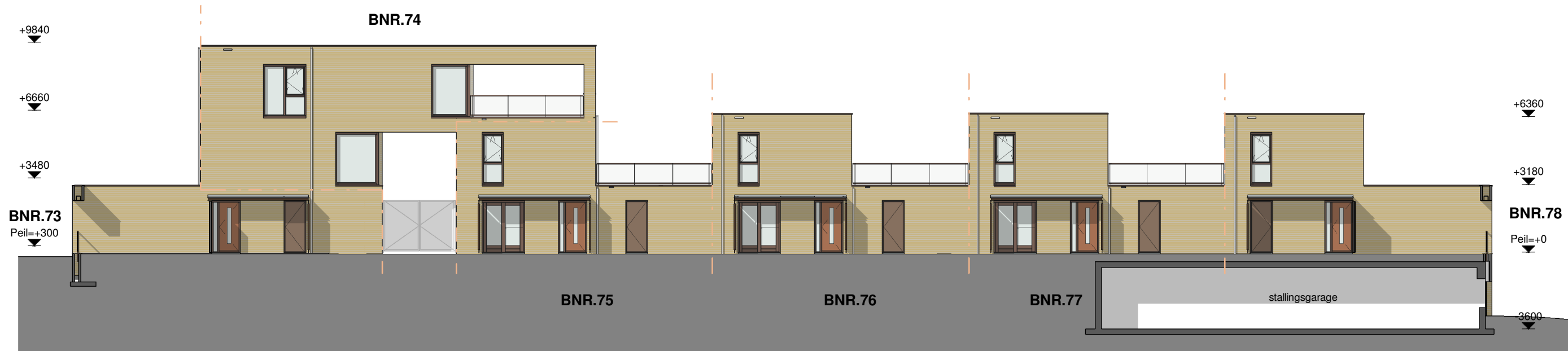
NOORDGEVEL BINNENHOF
