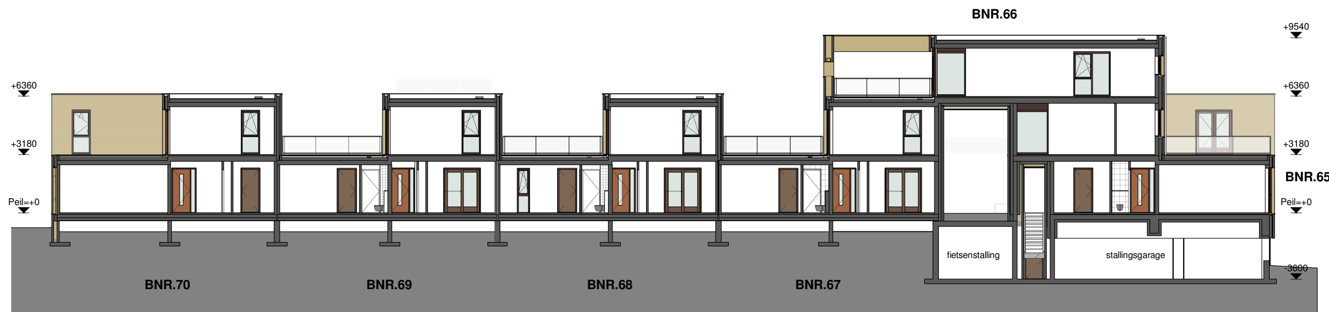
DOORSNEDE A-A
