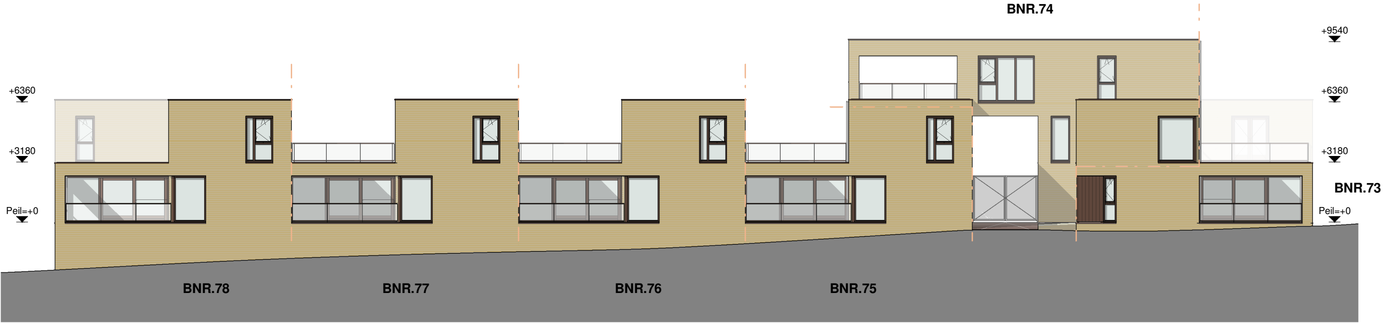
ZUIDGEVEL
