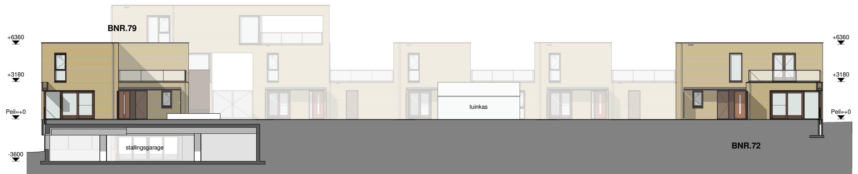
ZUIDGEVEL 2-KAPPER
