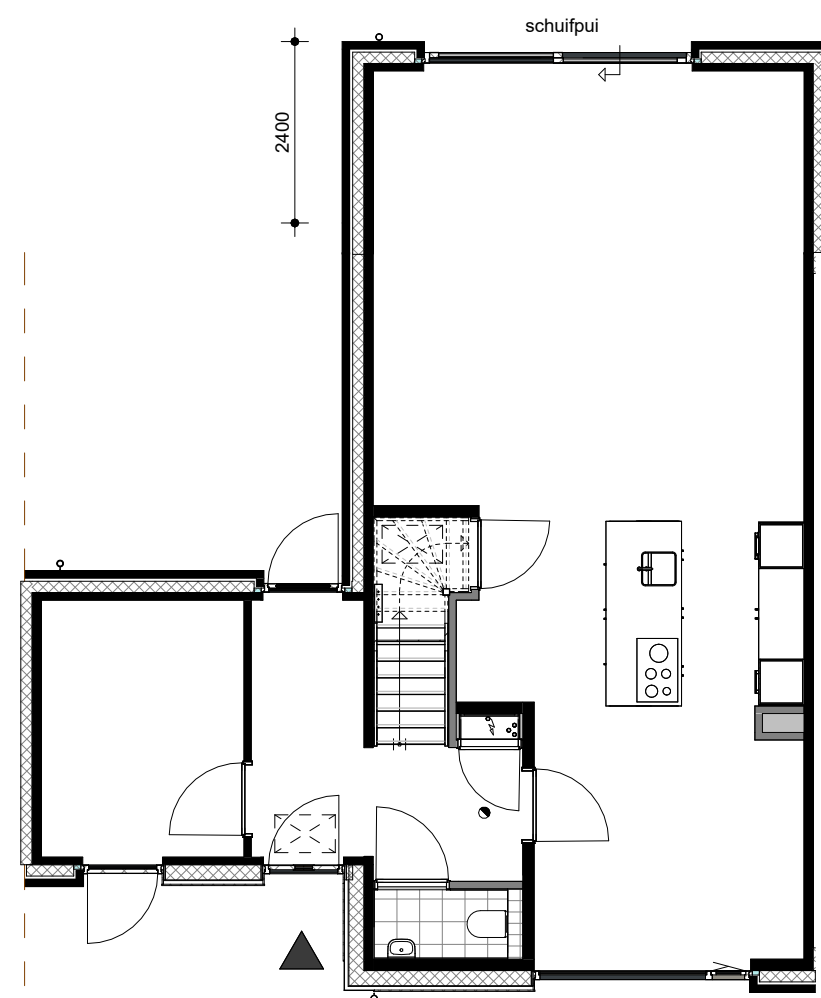
begane grond
