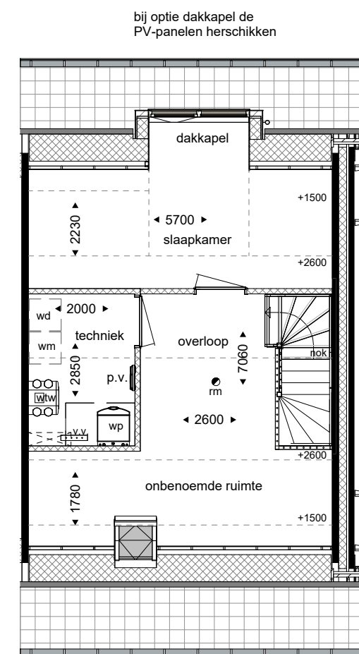
tweede verdieping
