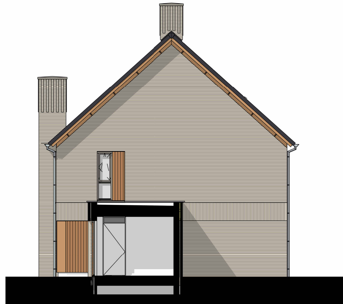
kavelnr: 63 rechter zijgevel
