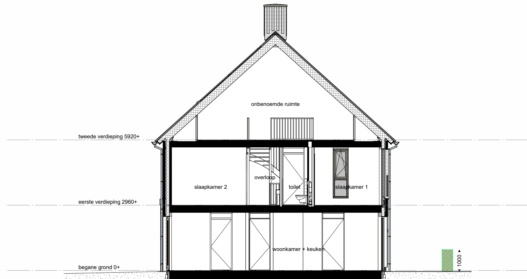
doorsnede
