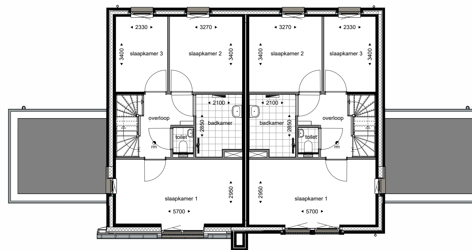
kavelnr: 64 kavelnr: 63 eerste verdieping
