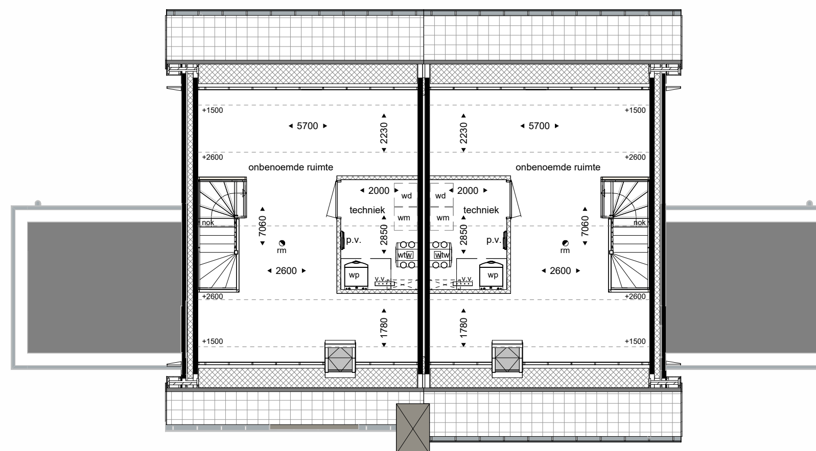
kavelnr: 64 kavelnr: 63 tweede verdieping
