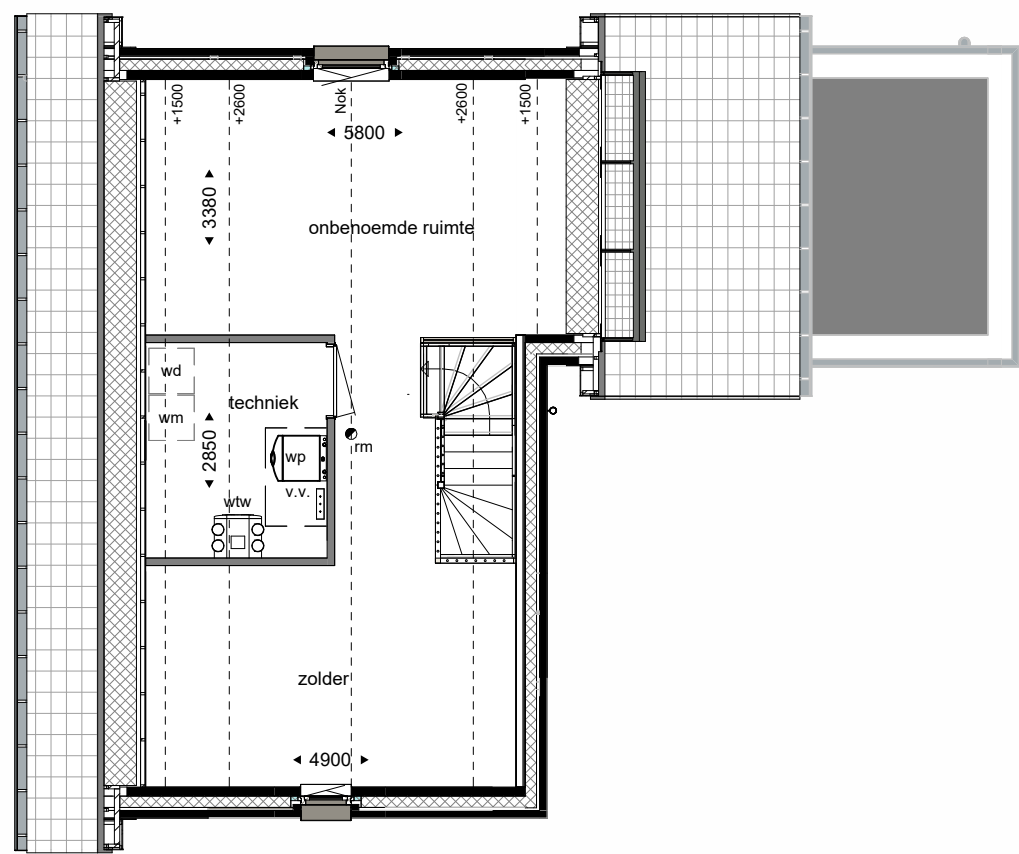
tweede verdieping
