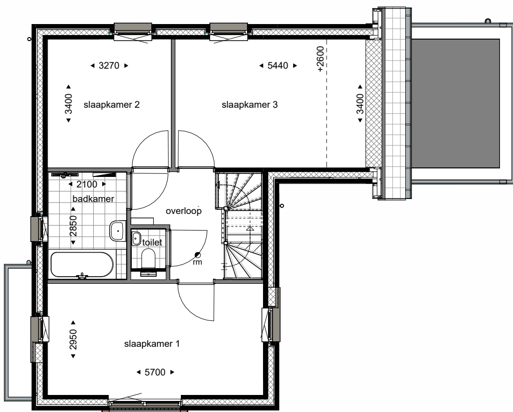
eerste verdieping
