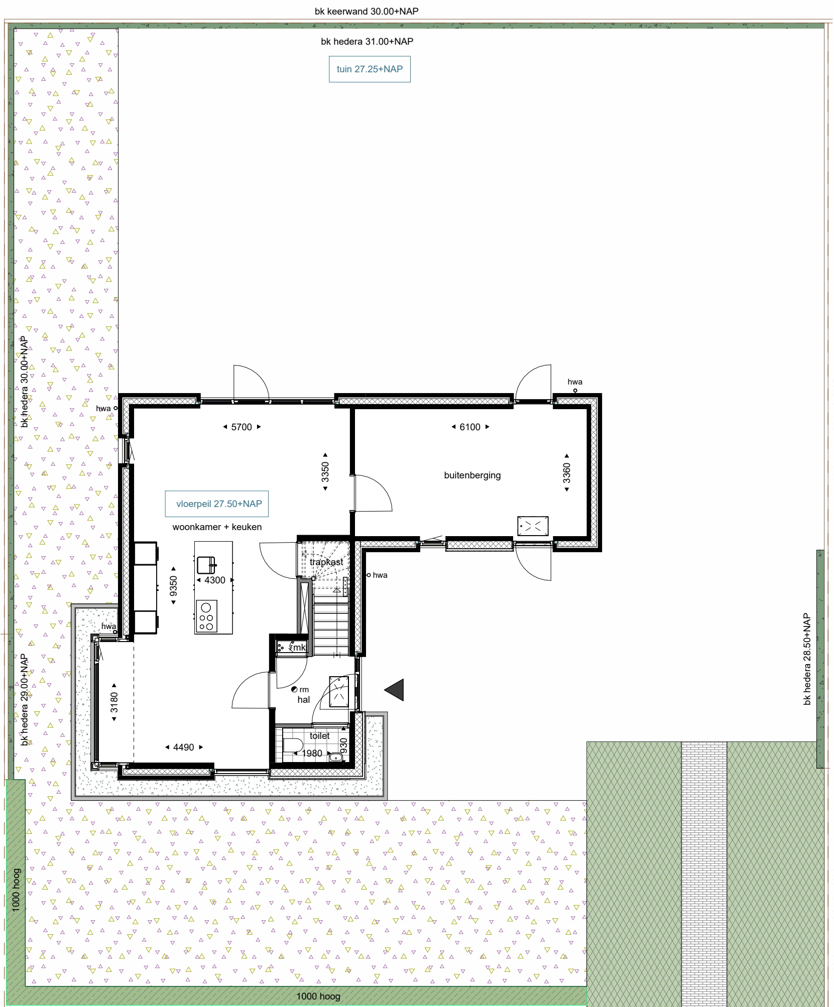
begane grond
