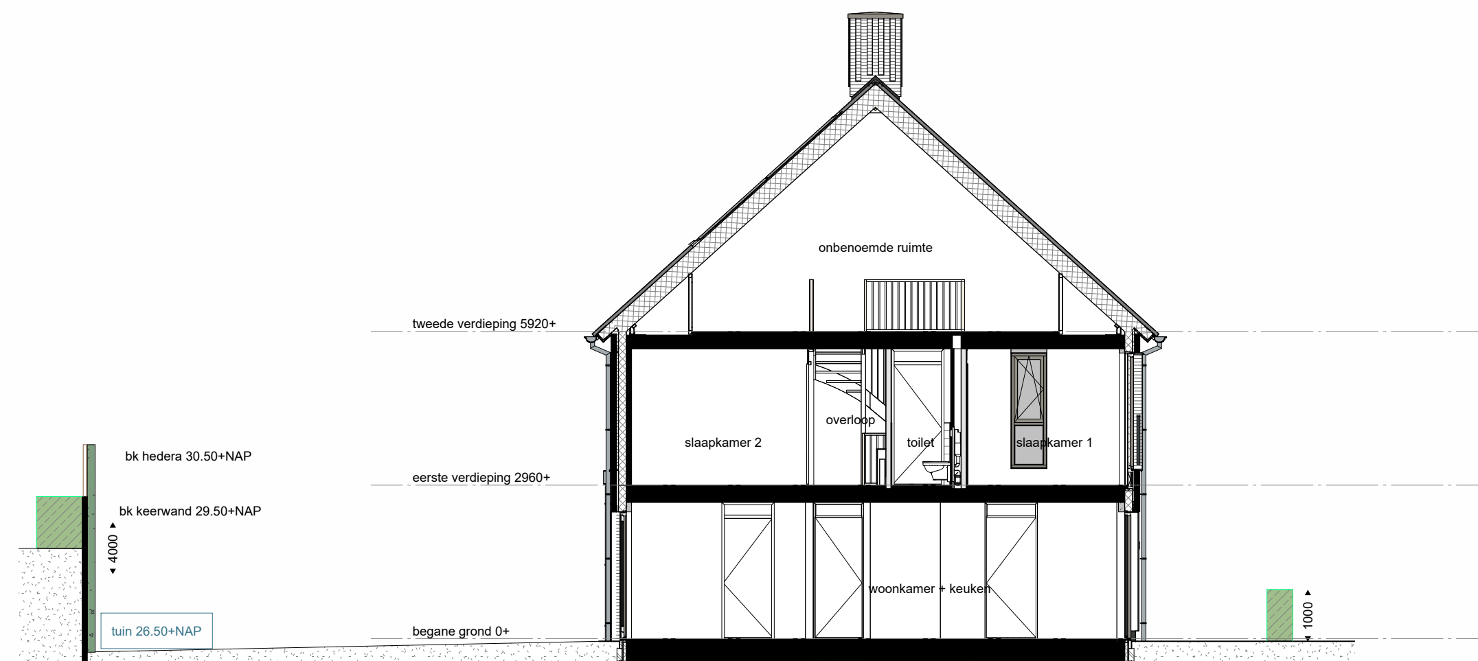
doorsnede
