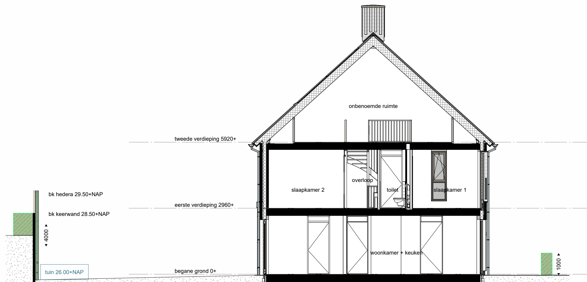
doorsnede
