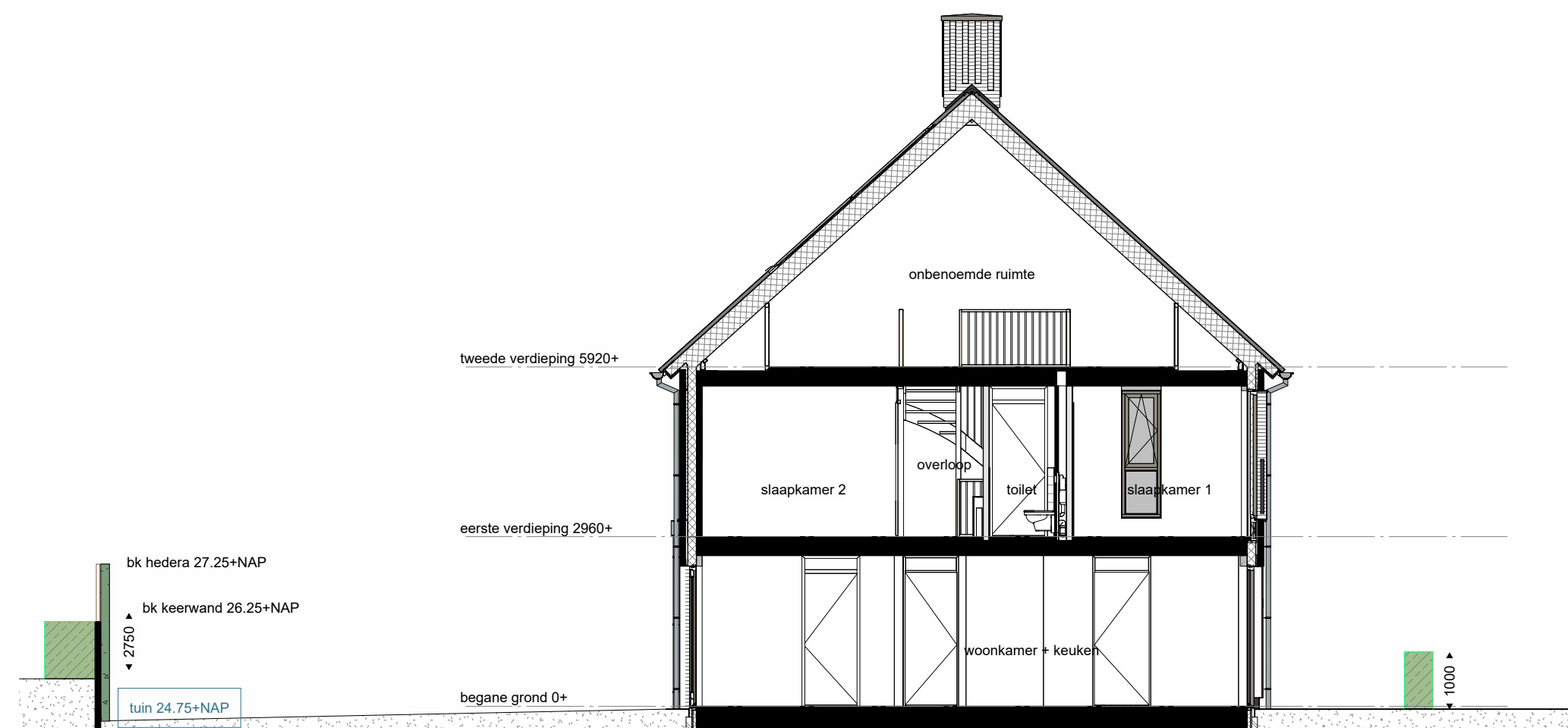
doorsnede
