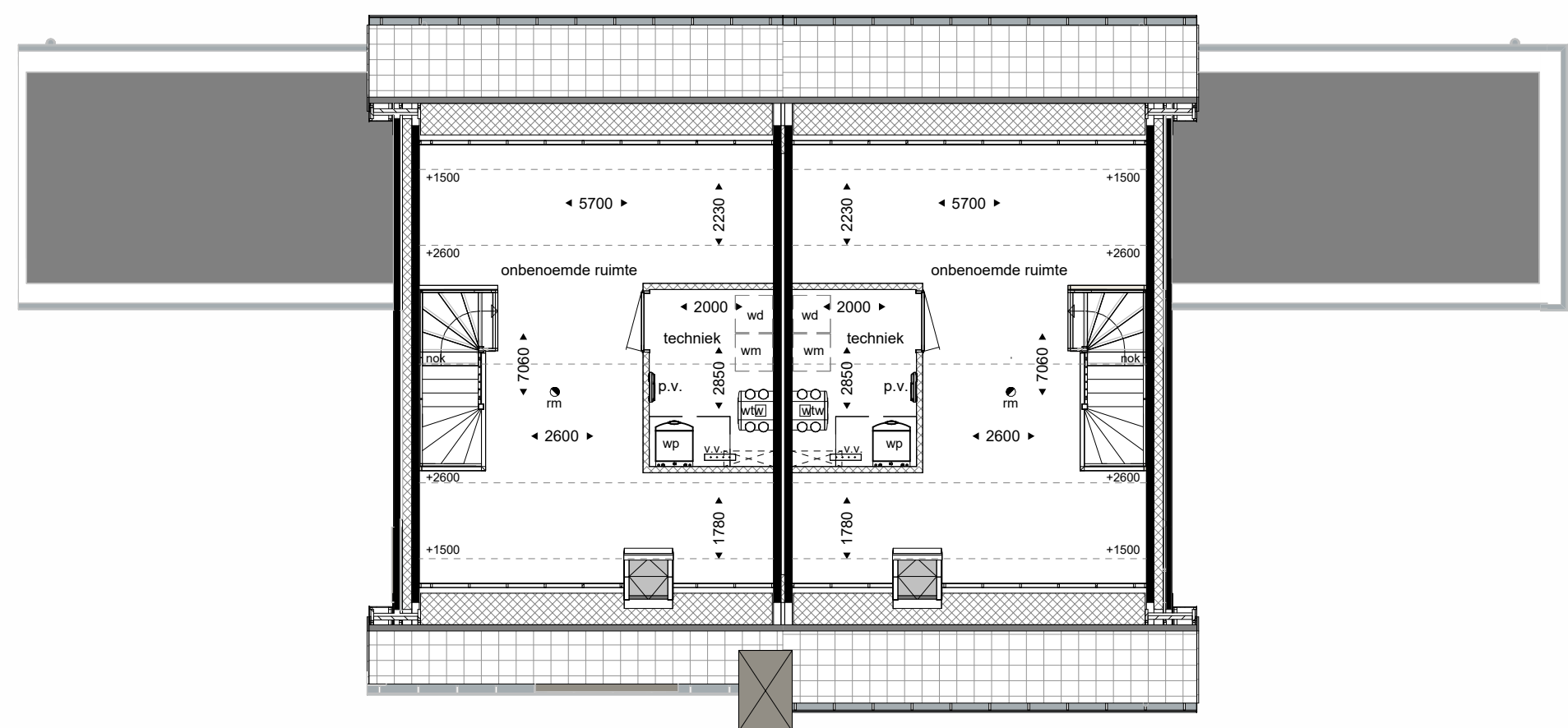
tweede verdieping
