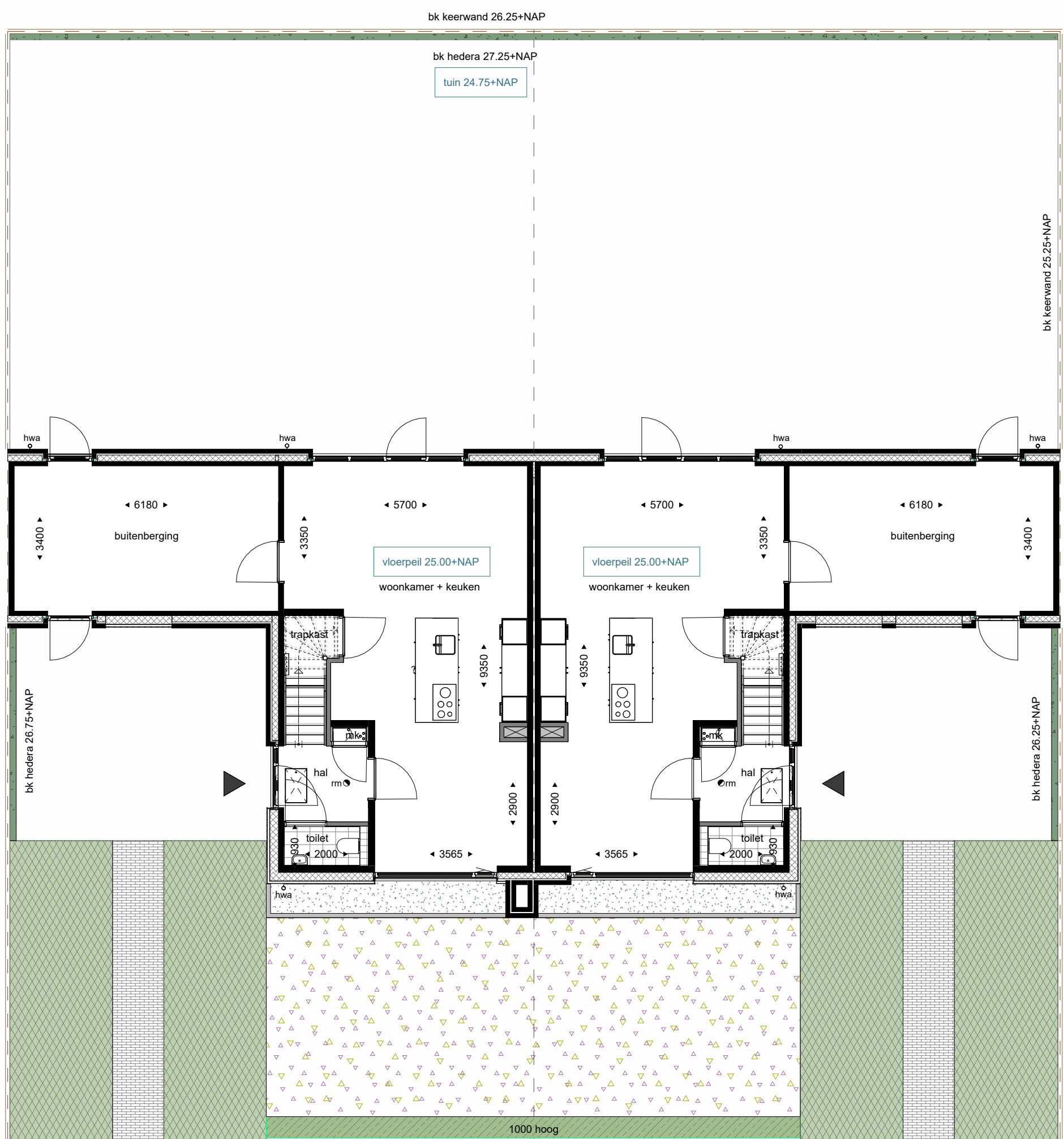
begane grond
