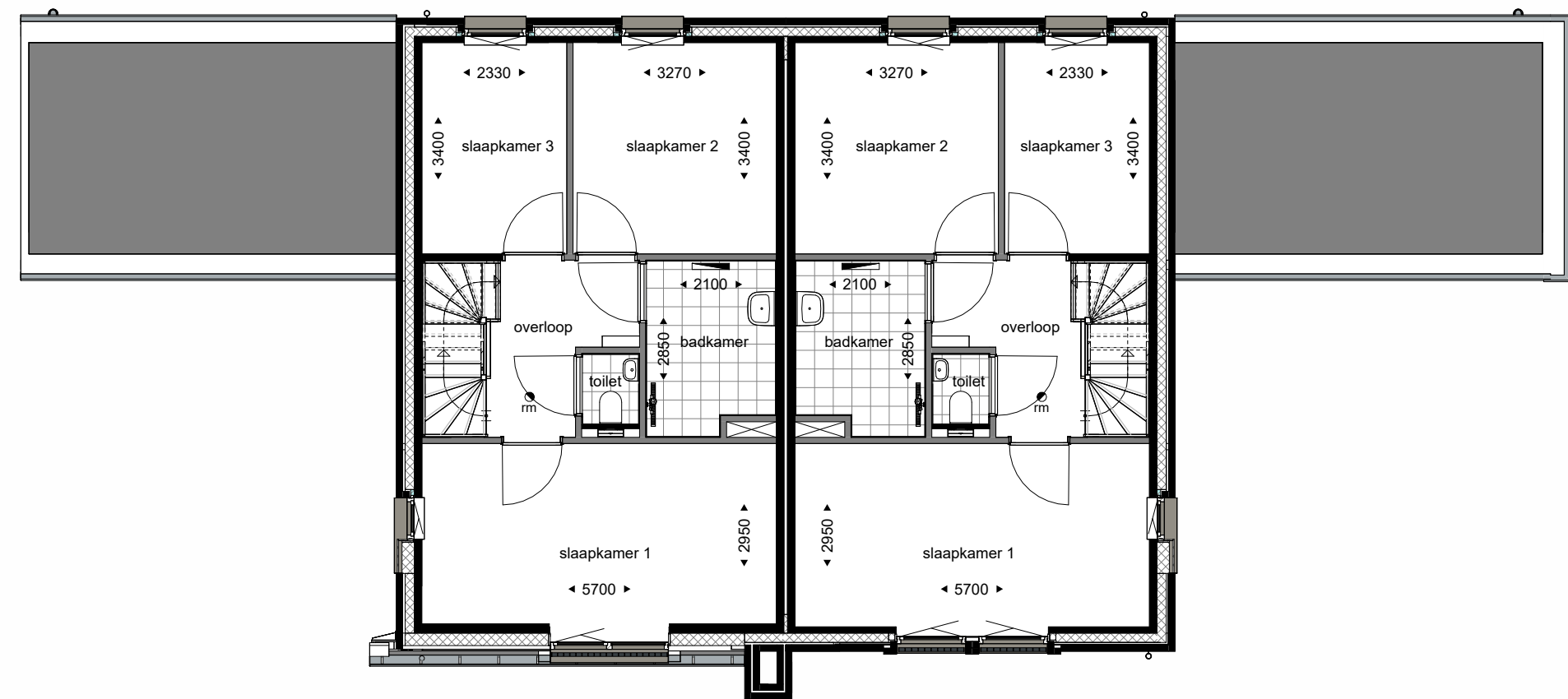
eerste verdieping
