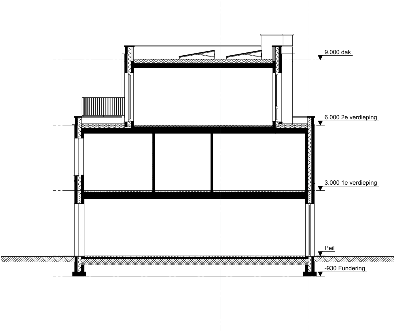
doorsnede
