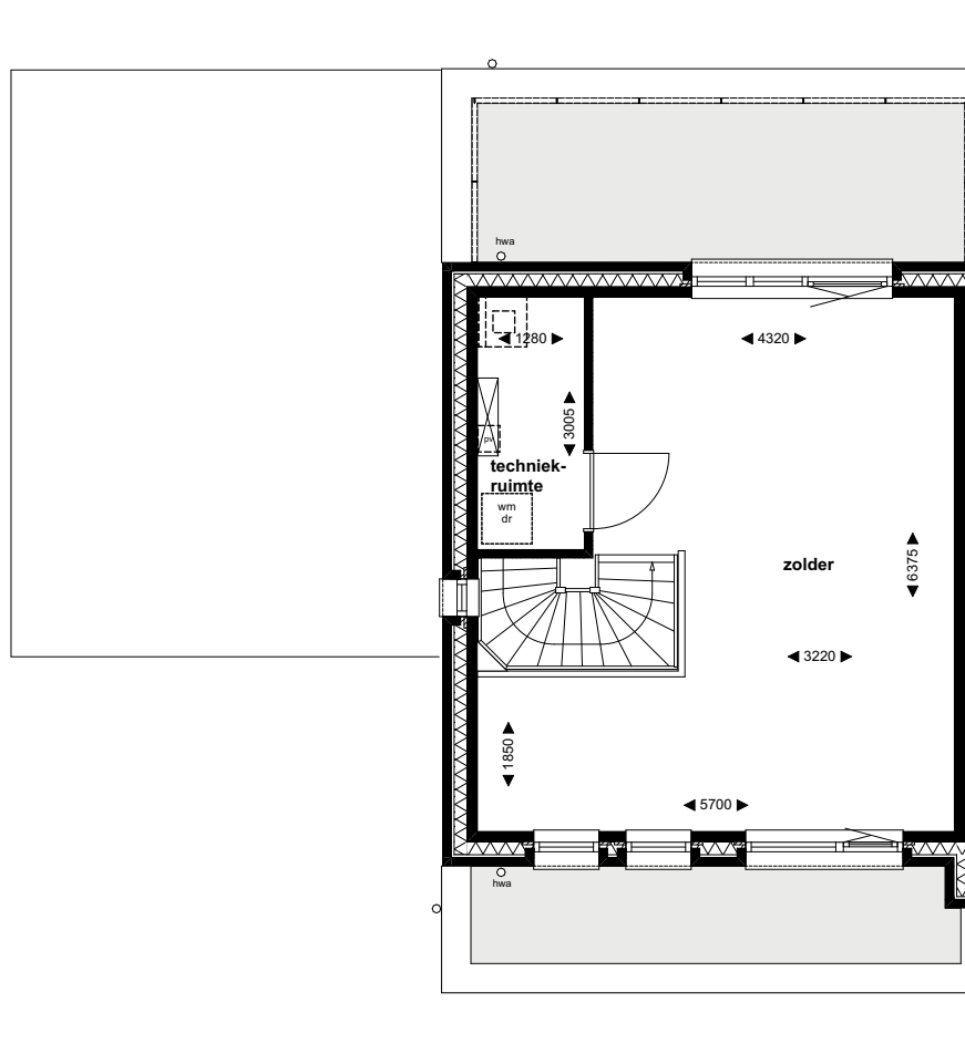
2e verdieping
