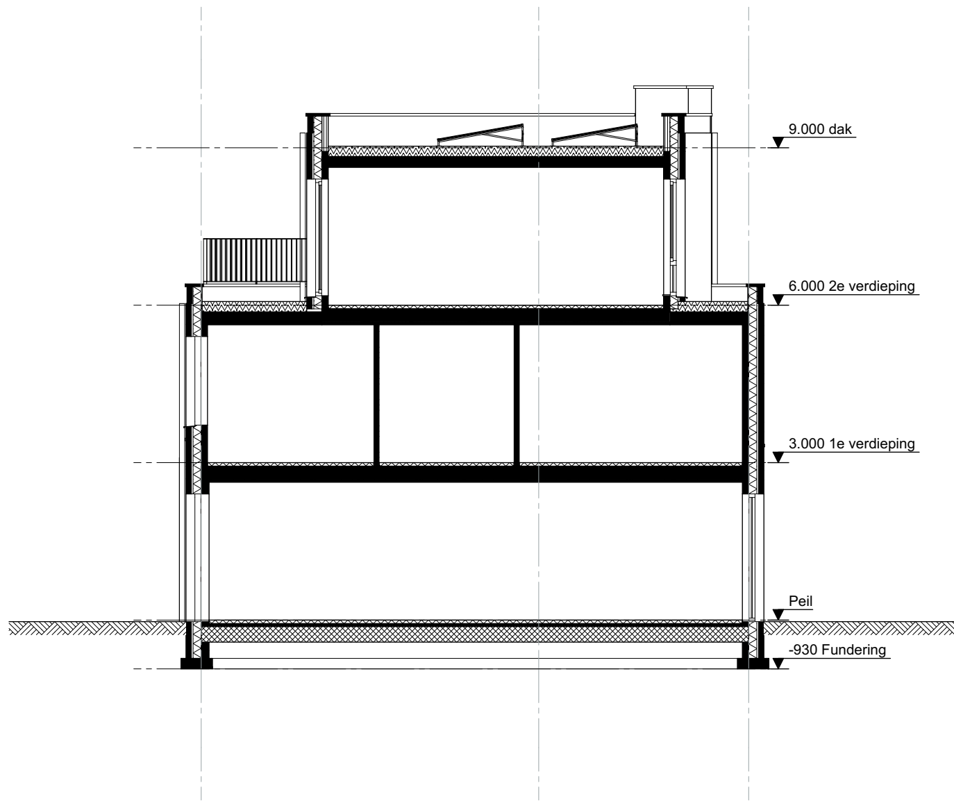
doorsnede
