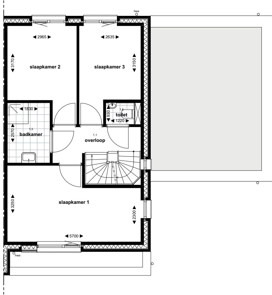
1e verdieping
