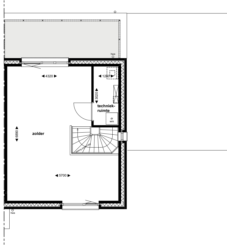
2e verdieping
