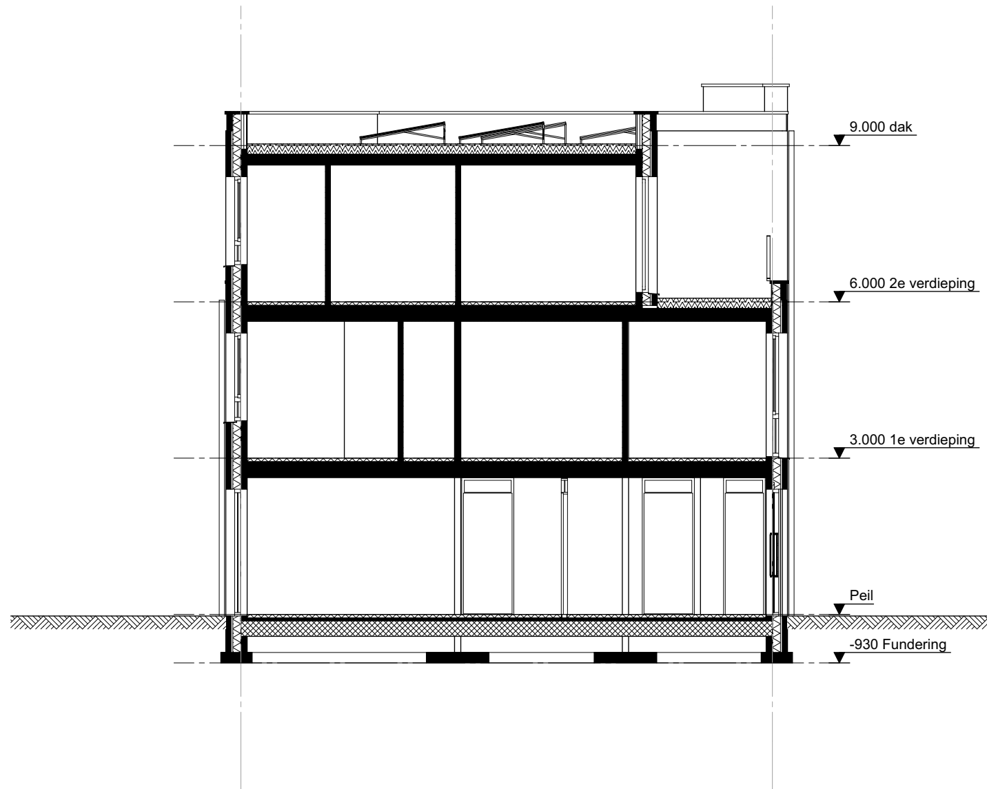
doorsnede
