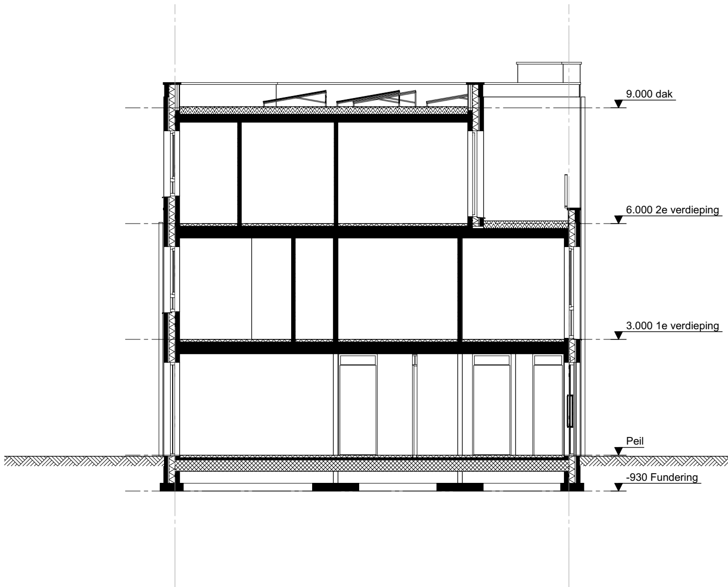
doorsnede
