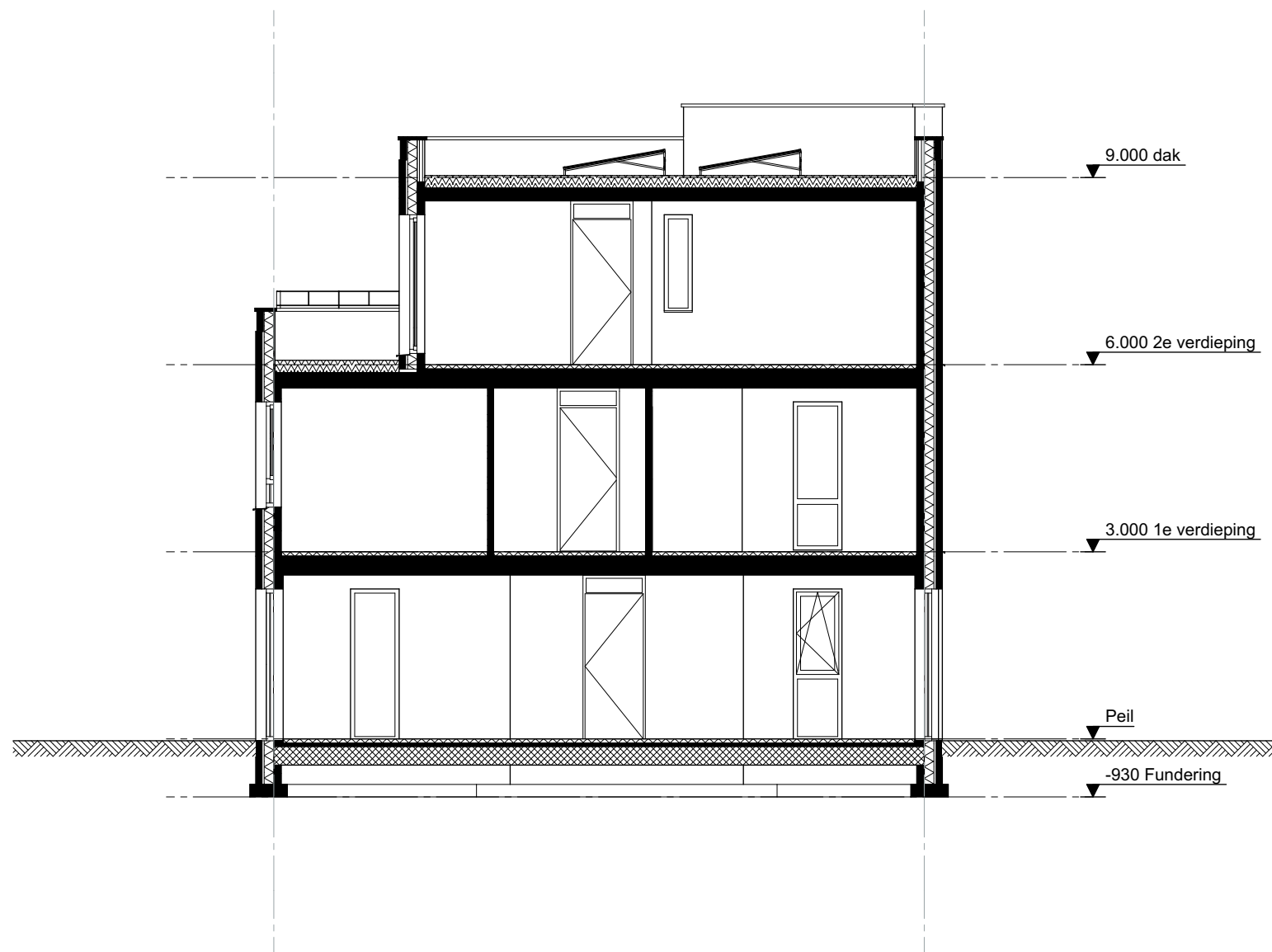
doorsnede
