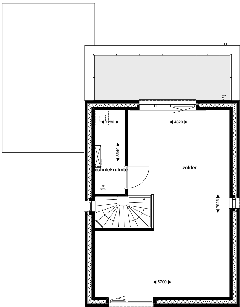
2e verdieping
