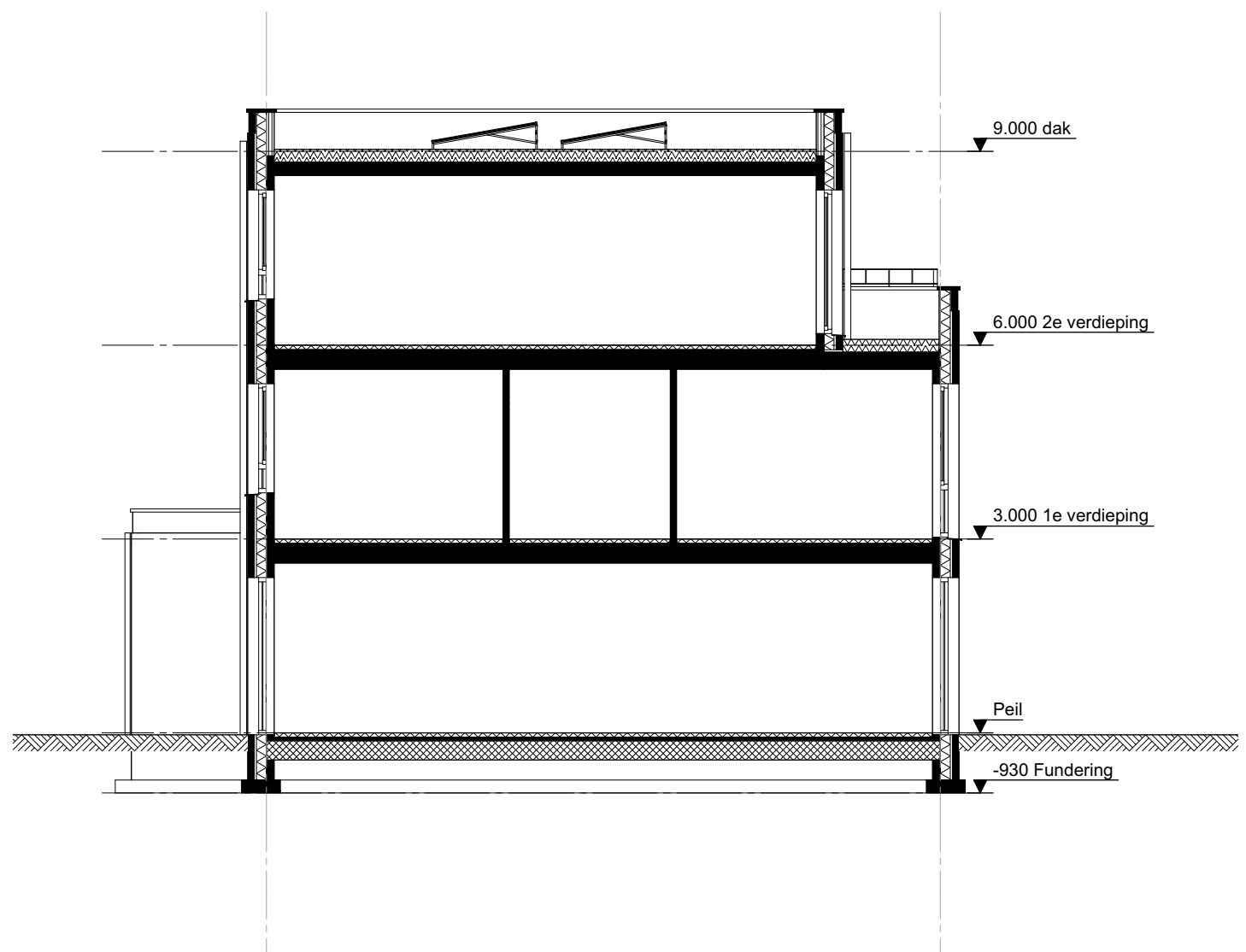
doorsnede
