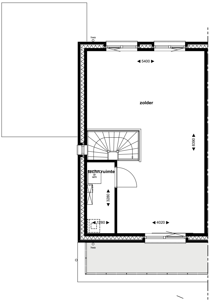
2e verdieping
