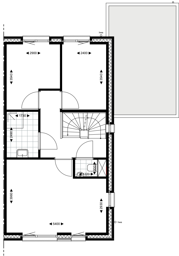
1e verdieping
