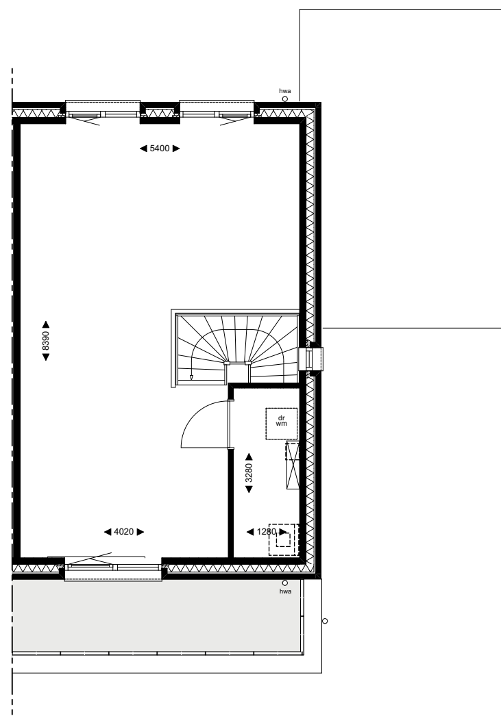
2e verdieping
