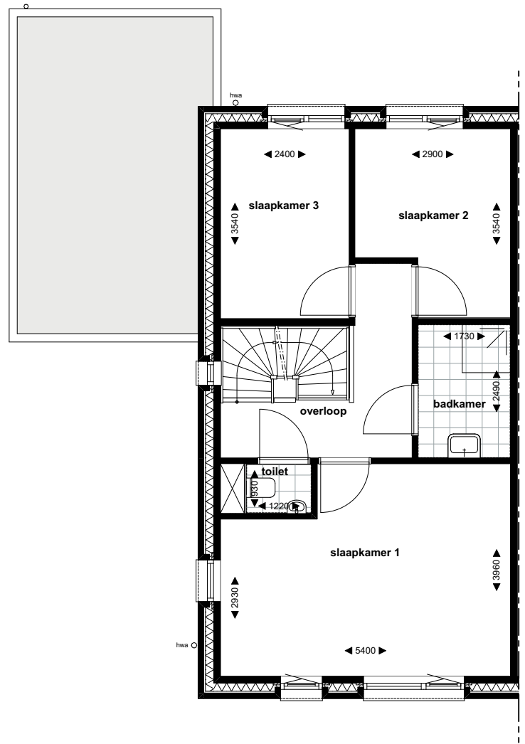
1e verdieping
