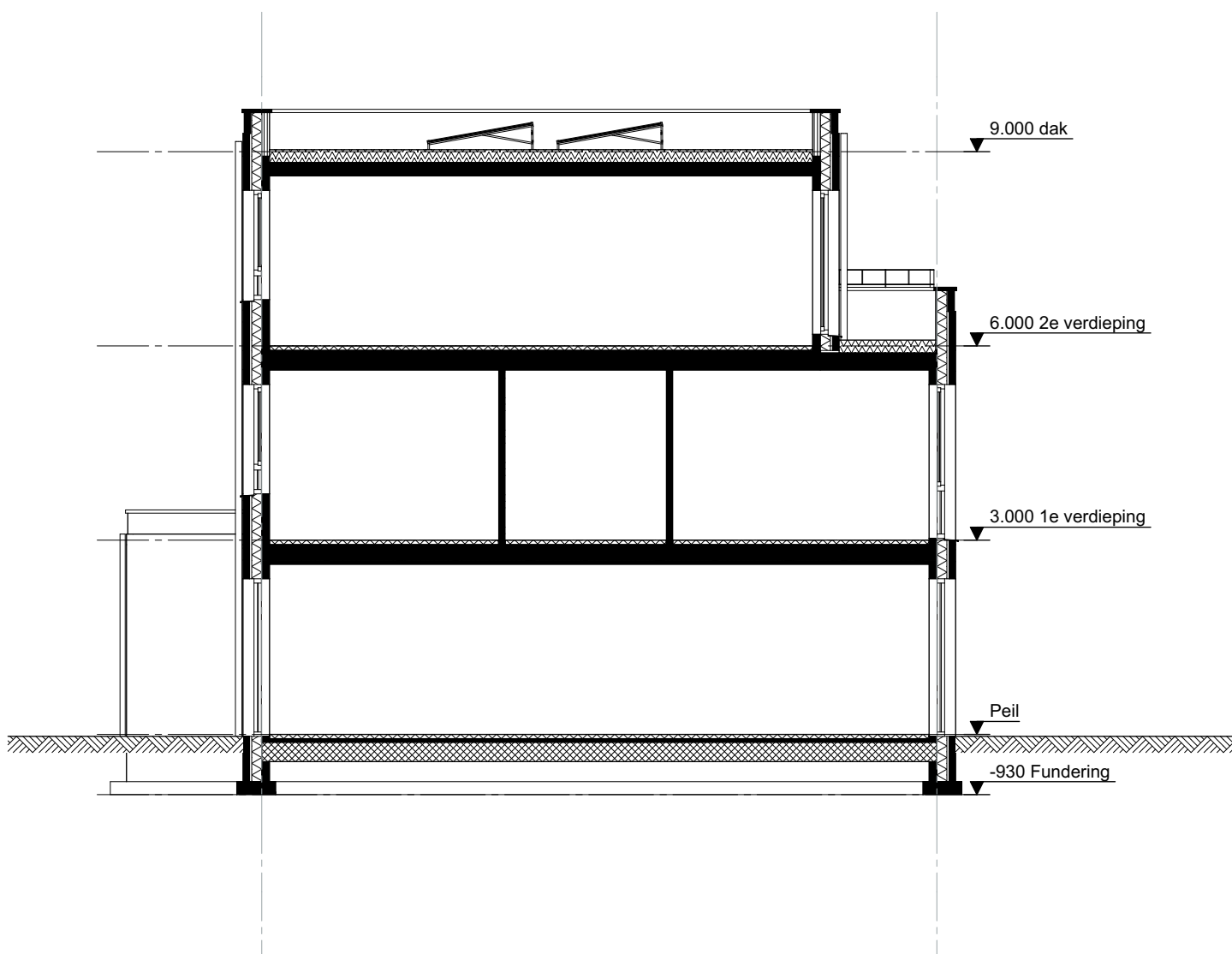
doorsnede
