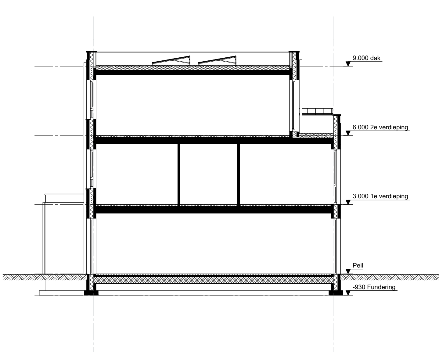
doorsnede
