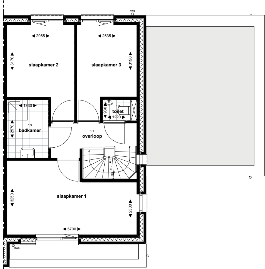
1e verdieping
