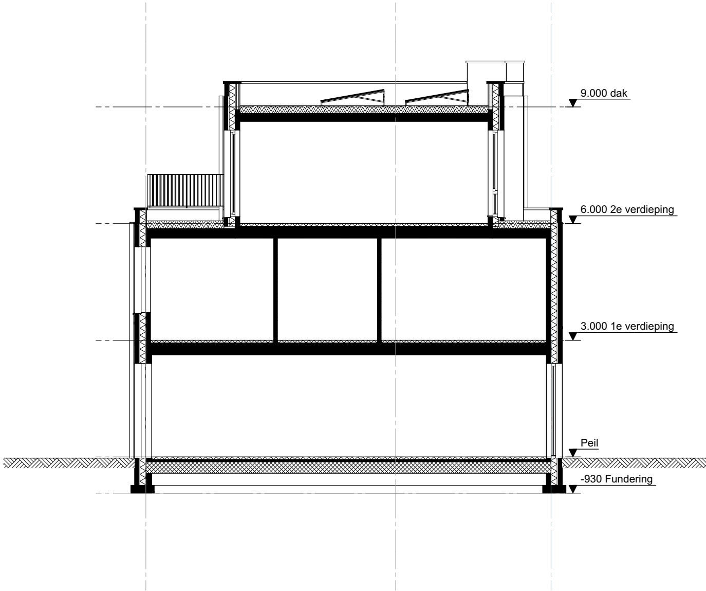
doorsnede
